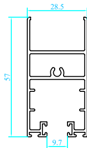
Thanh ngang dưới cửa đi trượt LW
