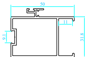
Thanh đứng móc phải cửa đi trượt LW
