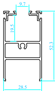
Thanh ngang trên cửa đi trượt LW
