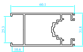
Thanh đứng trơn cửa đi trượt LW
